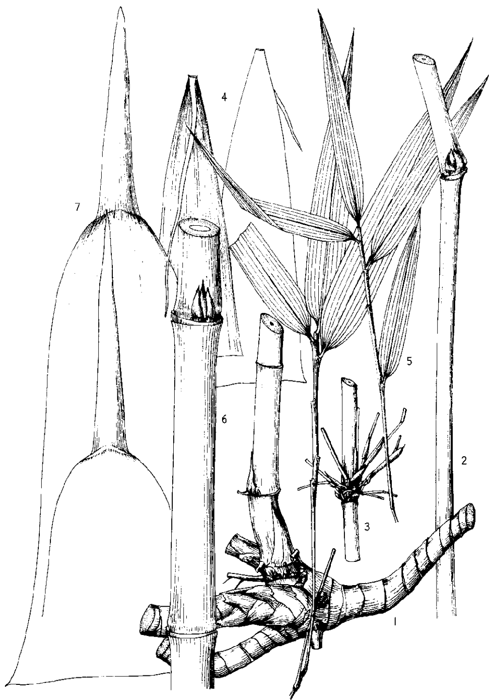
图版 109 1-5. 扫把竹 Fargesia fractiflexa Yi: 1. 地下茎及竿之基部; 2. 竿之一段, 示笋芽; 3. 竿之一段, 示分枝; 4. 竿箨; 5. 具叶小枝。6-8. 窝竹 Fargesia brevissima Yi: 6. 竿之一段, 示短而中空之节间; 7. 竿箨; 8. 具叶小枝。(杨林绘)
