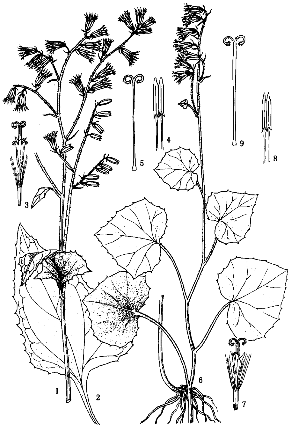
图版 11 1—5. 丽江蟹甲草 Parasenecio lidjiangensis (Hand.-Mazz.) Y. L. Chen: 1, 2. 植株; 3. 小花; 4. 花药; 5. 花柱分枝。6—9. 大理蟹甲草 P. taliensis (Franch.) Y. L. Chen: 6. 植株; 7. 小花; 8. 花药; 9. 花柱分枝。(张春芳绘)
