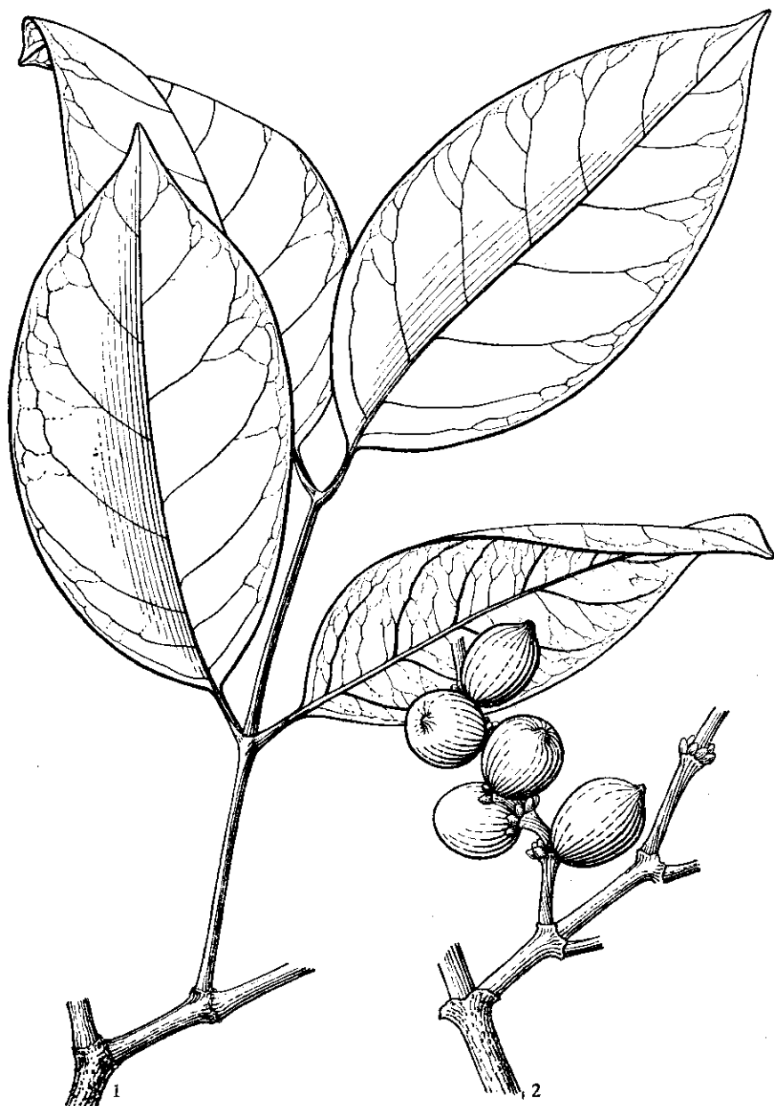
海南买麻藤 Gnetum hainanense C. Y. Cheng. 1. 枝及叶; 2. 成熟雌球花序的一部分及种子。 (张泰利绘)
