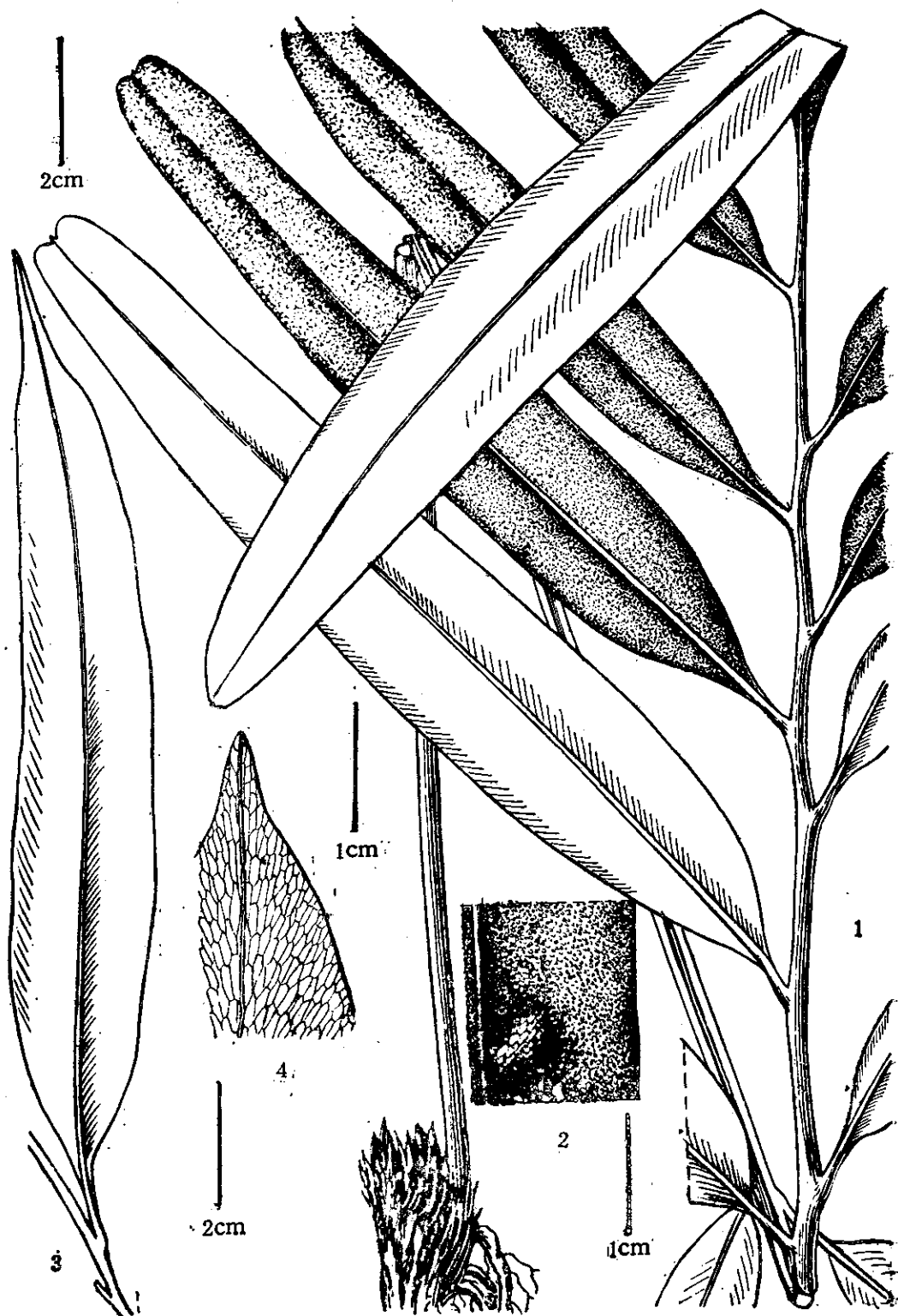
1—2. 鹼蕨 Acrostichum aureum L.: 1. 植株全形, 2. 能育羽片的一部分(放大)。3—4. 尖叶鹼蕨 Acrostichum speciosum Willd.: 3. 一片不育羽片, 4. 不育羽片的顶部(放大)。(张荣厚绘)
