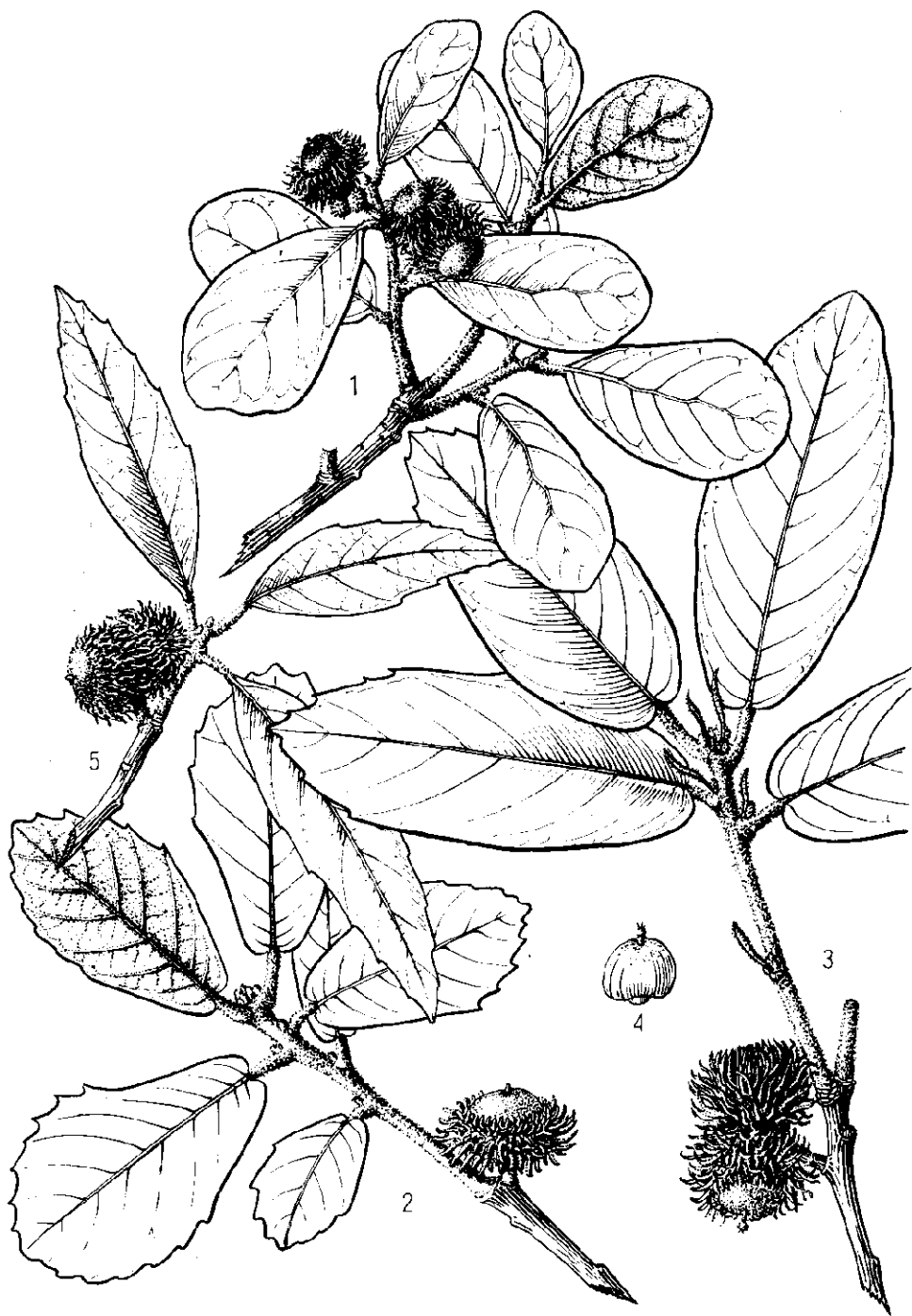
图版 77 1. 长苞高山栎 Quercus fimbriata Chun et Huang: 果枝。2. 匙叶栎(原变种) Q. dolicholepis A. Camus var. dolicholepis : 果枝。3—4. 尖叶栎 Q. oxyphylla (Wils.) Hand.-Mazz.: 3. 果枝, 4. 坚果。5. 橐子栎(原变种) Q. baronii Skan var. baronii : 果枝。(余汉平绘)
