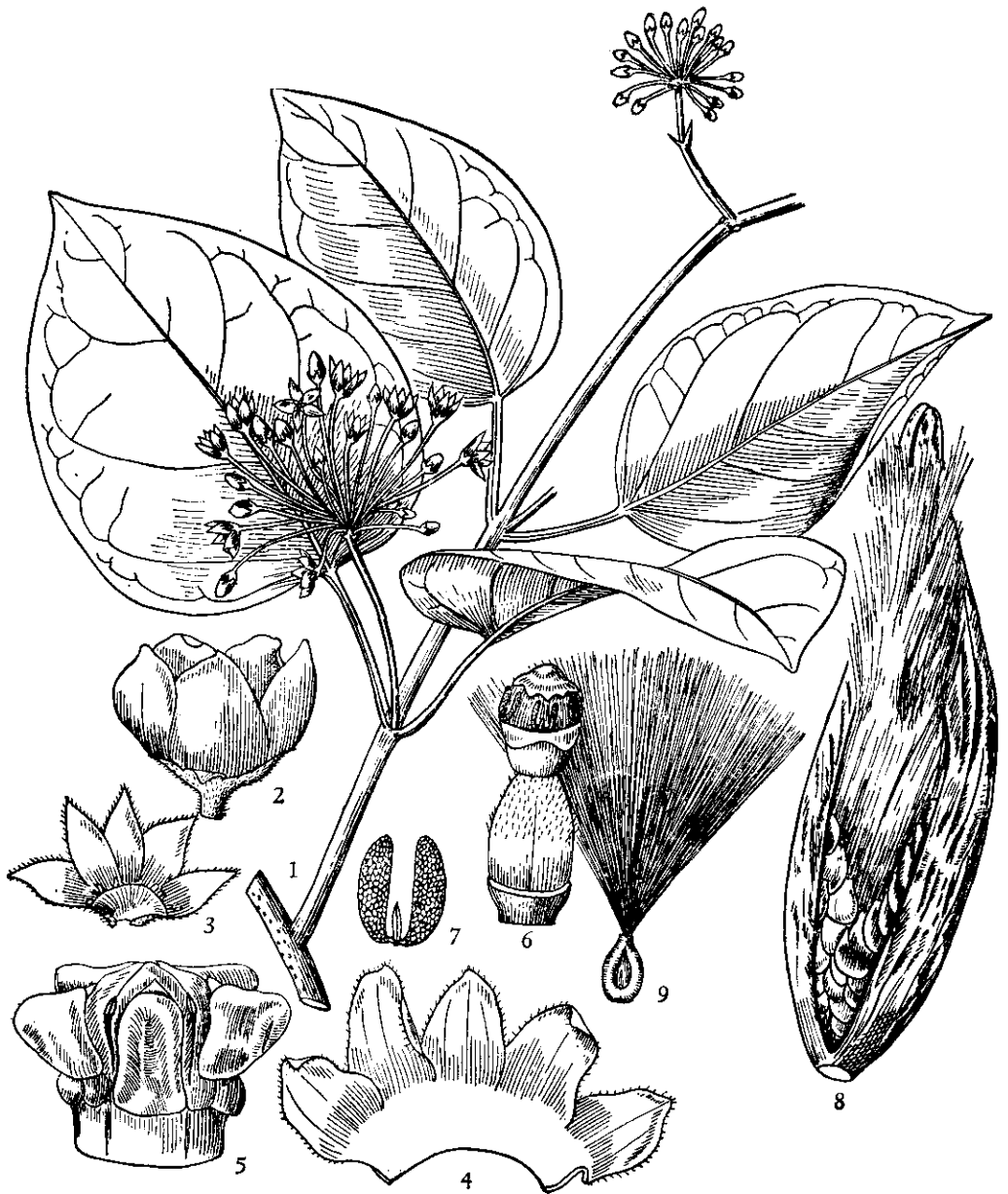
图版 183 南山藤 Dregea volubilis (L. f.) Benth. ex Hook. f., 1.花枝; 2.花; 3.花萼展开示腺体; 4.花冠展开; 5.合蕊柱和副花冠; 6.雌蕊; 7.花粉器; 8.蓇葖; 9.种子。(陈国泽仿绘)
