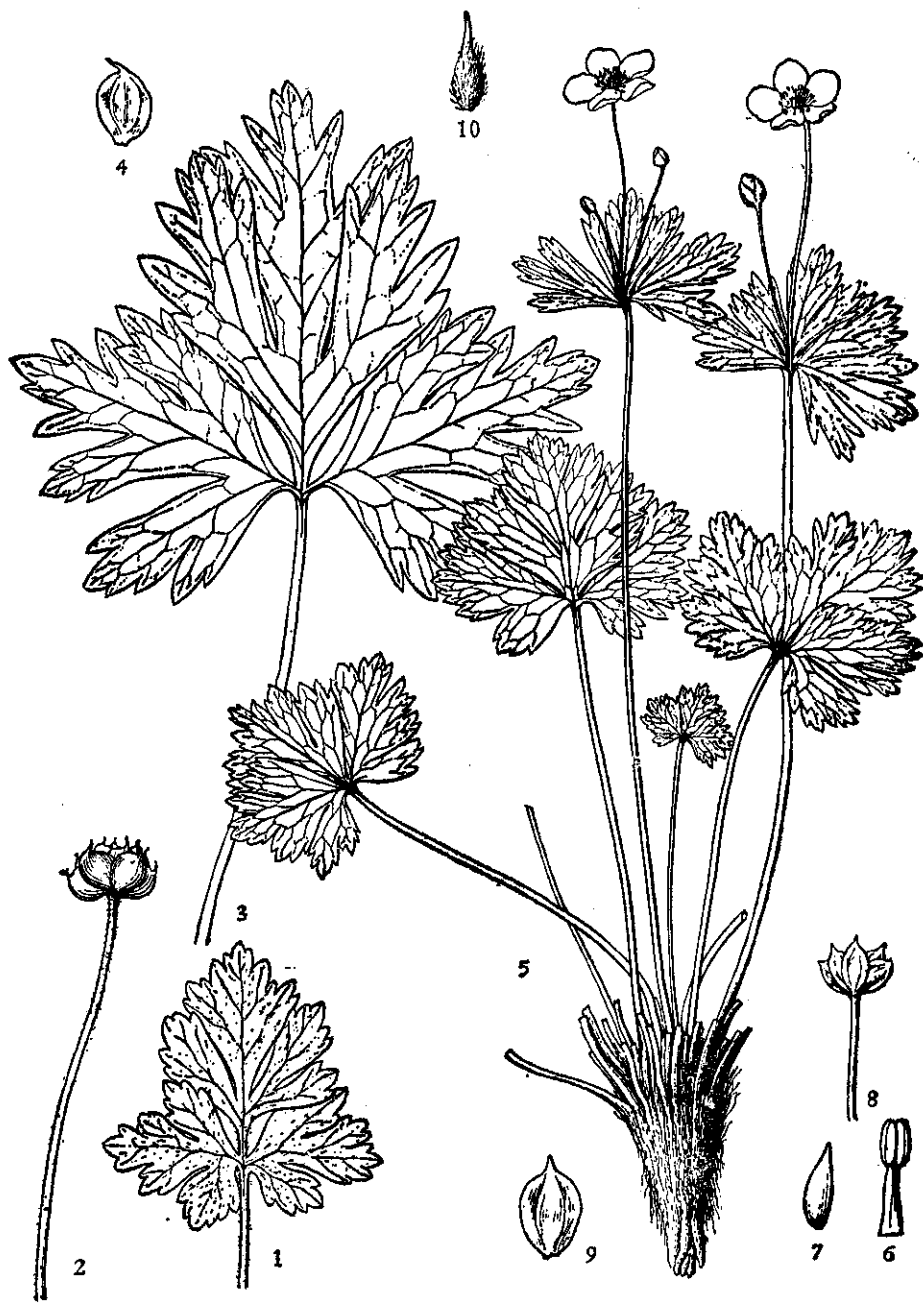
1—2. 云南银莲花 Anemone aemissa var. yunnanensis 1. 基生叶; 2. 聚合果。3—4. 太白银莲花 A. taipaiensis 3. 基生叶; 4. 瘦果。5—9. 银莲花 A. cathayensis 5. 植株全形; 6. 雄蕊; 7. 心皮; 8. 聚合果; 9. 瘦果。10. 毛蕊银莲花 A. cathayensis var. hispida 10. 心皮。
