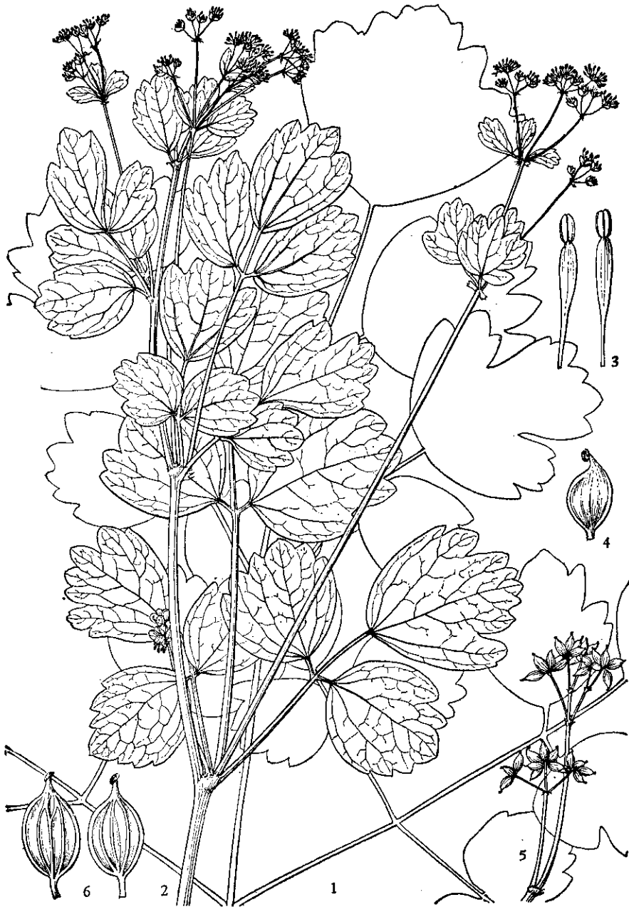
1—6 贝加尔唐松草 Thalictrum baicalense 1. 基生叶的一部分; 2. 植株上部; 3. 雄蕊; 4. 心皮; 5. 果序; 6. 瘦果。(史涓清绘)
